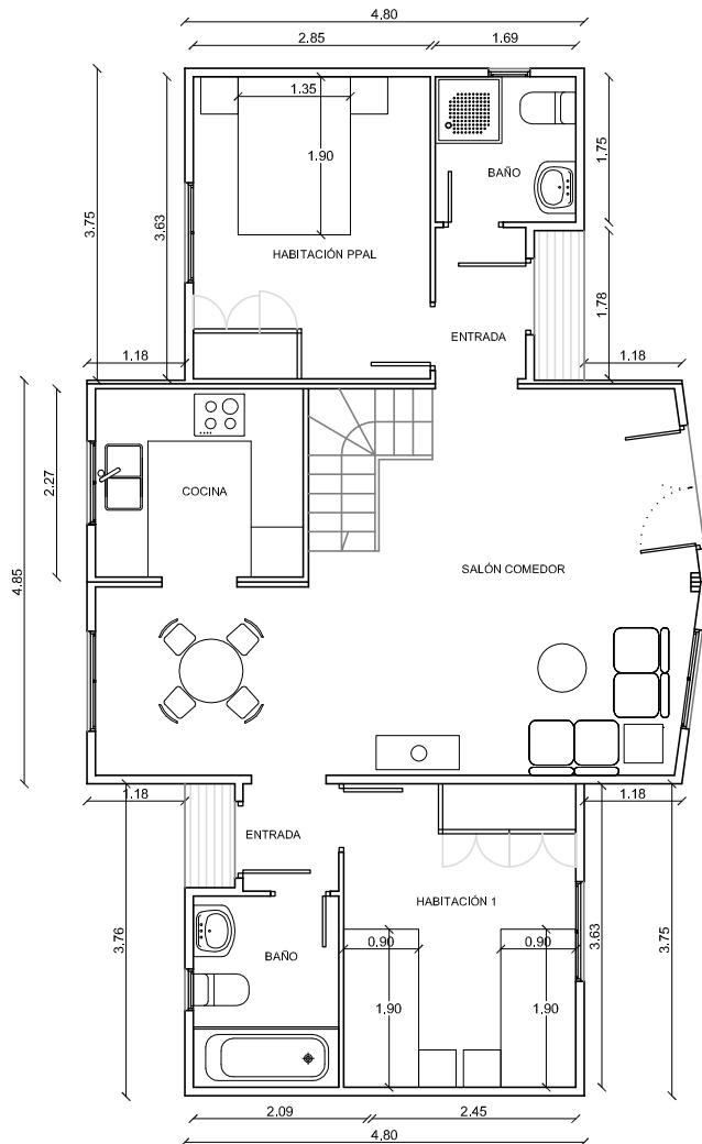
PLANTA BAJA SUPERFICIE VIVIENDA: 96 m 2
